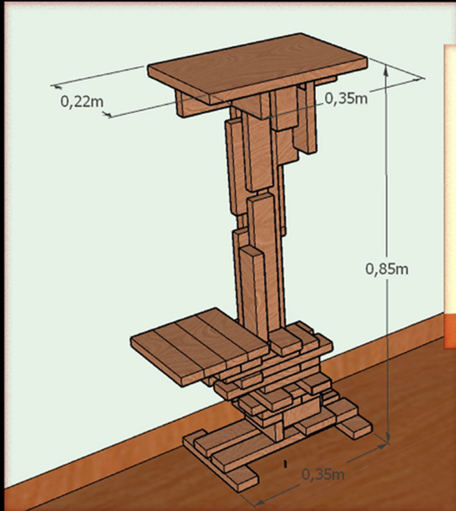
DIMENSIONES BASICAS
