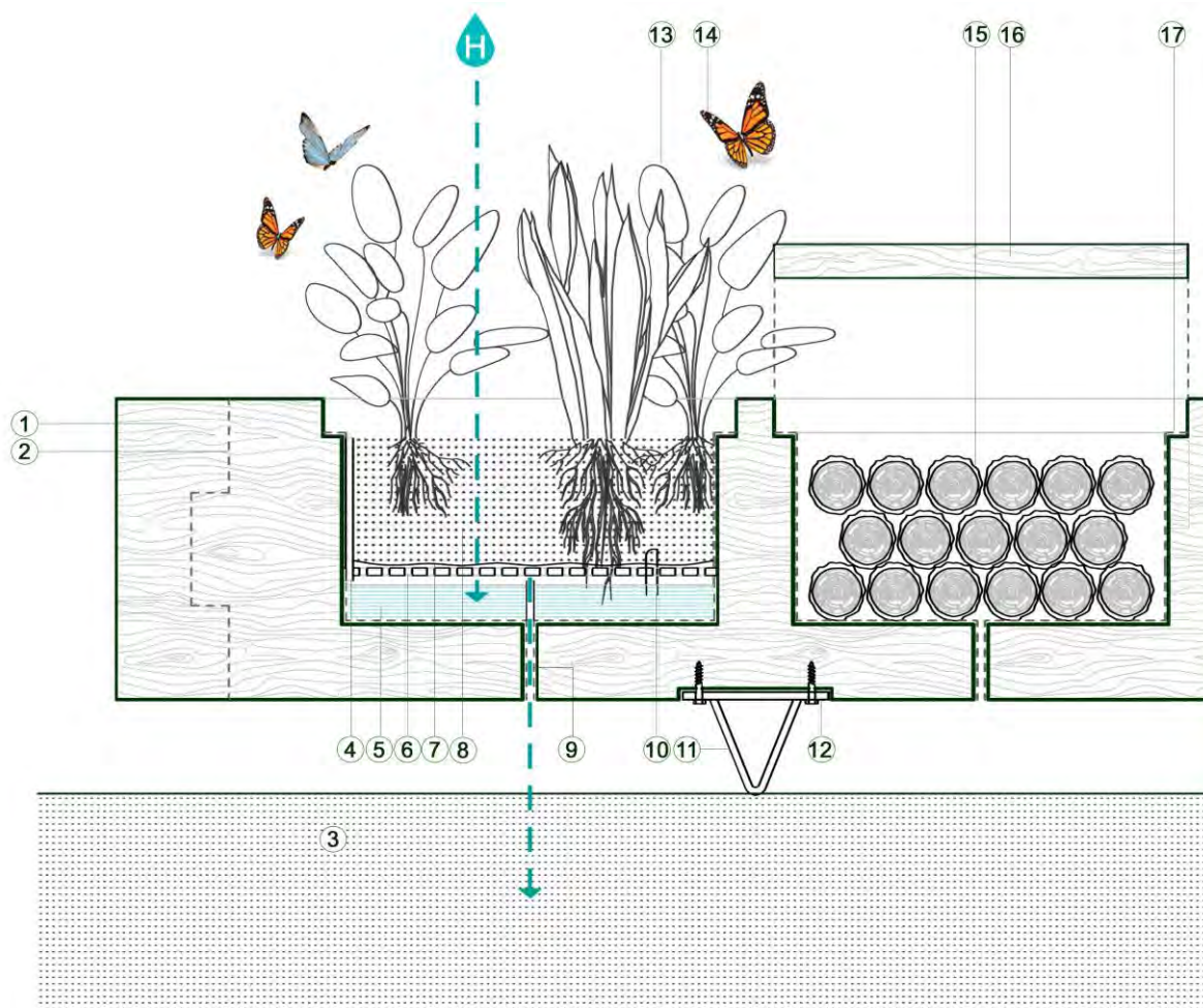
Detalle constructivo 1/5
